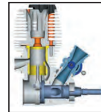
Top Dead Center
