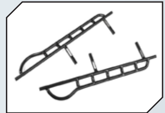
Art.Nr.: RC4ZS2132 RC4WD Tough Armor Steel Side Sliders für Jeep JT
