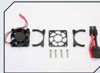
Art.Nr.: GPMSLA018FANLCGBK GPM Aluminium Motor Kühlkörper mit Ventilator schwarz
